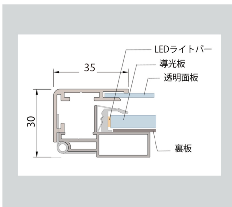
アルミフレーム断面略図
